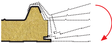
Sistema de montaje de los paneles Isofire Roof
